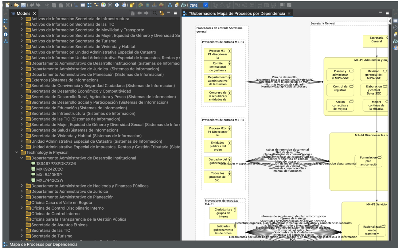
Figura 2. Muestra Repositorio Archimate
